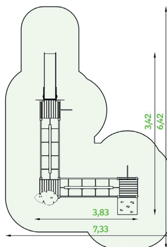
Rzut urządzenia wraz ze strefą funkcjonalną
